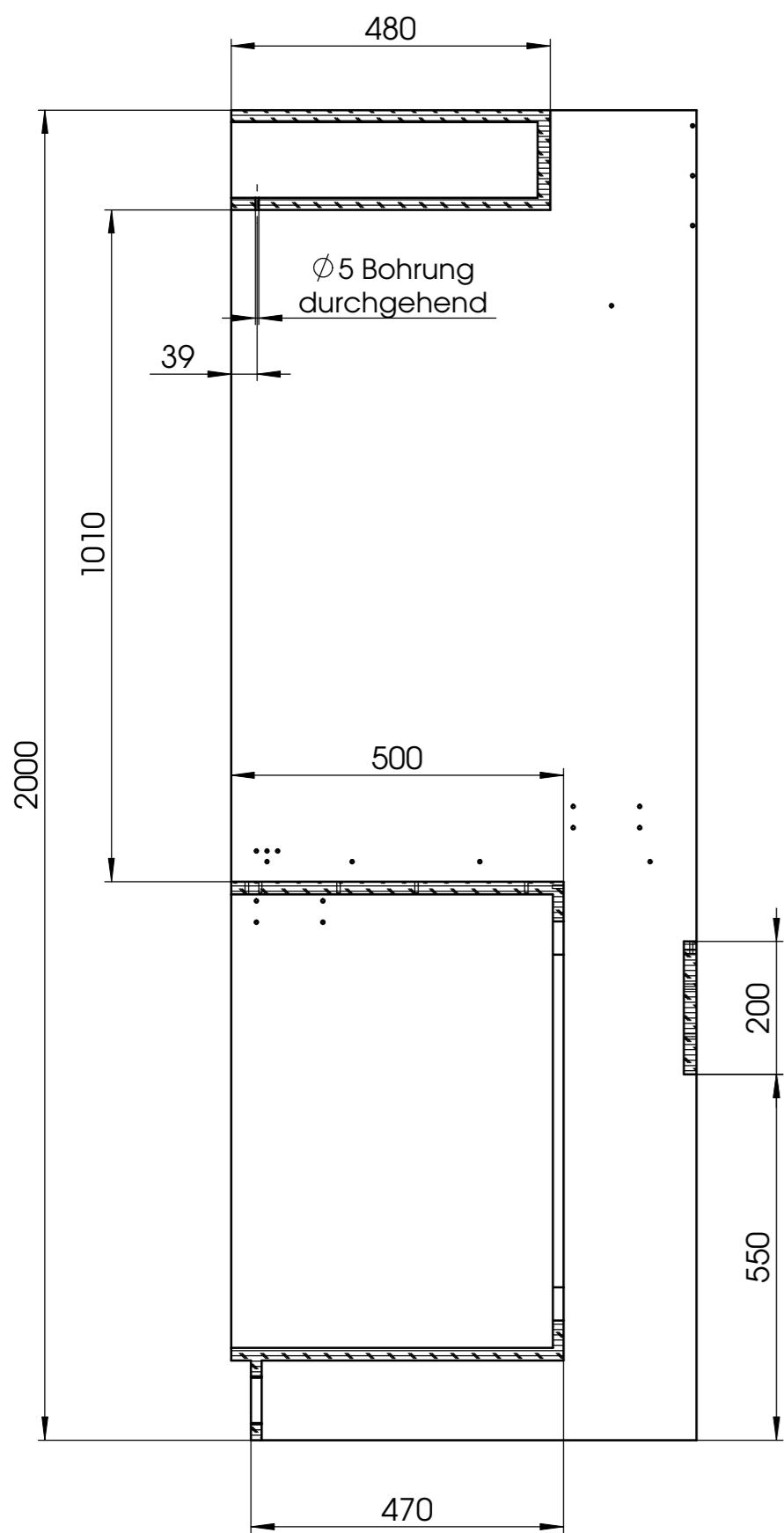
Schnitt A-A
