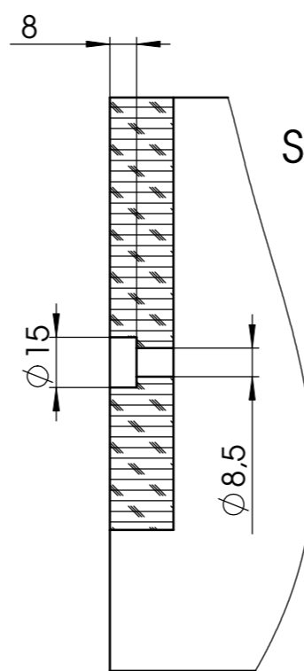
Schnitt B-B
